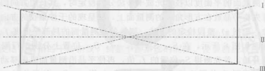
图 7 光隙法检定刀口形直尺的检定方位
