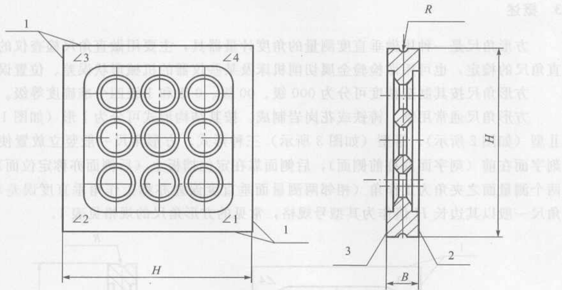
图 3 III 型方形角尺
